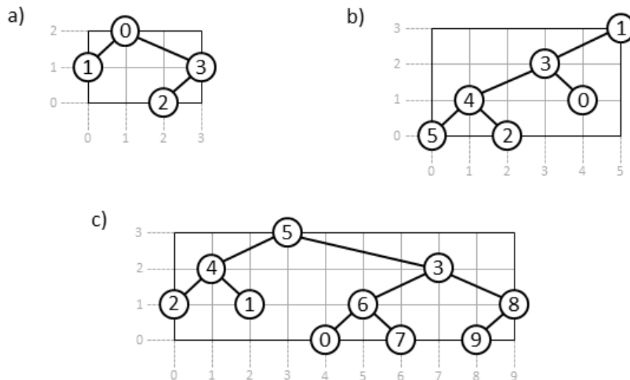
Obrázek 5: Příklady vizualizací binárních stromů ve čtvercové mřížce. Rozměry mřížek jsou a) 3 \times 4 , b) 4 \times 6 , c) 4 \times 10 .
