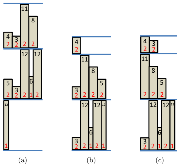
Obrázek 11: Abecedně seřazené knihy mají rozměry (výška \times tloušťka): 4 \times 2 , 3 \times 2 , 11 \times 2 , 8 \times 2 , 5 \times 2 , 3 \times 2 , 12 \times 2 , 6 \times 1 , 12 \times 2 , 12 \times 1 . Délka police je L = 9 . (a) Rozmístěný podle naivního algoritmu s cenou 11 + 12 + 12 = 35 . (b) Řešení s cenou 4 + 11 + 12 = 27 a maximální mezerou 7. (c) Optimální řešení s cenou 27 a minimální maximální mezerou 5.
