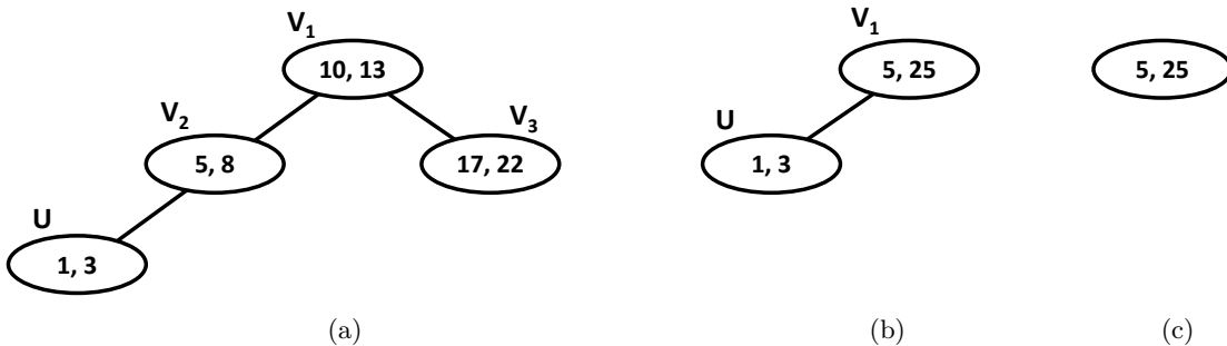
Obrázek 9: a) Stav původně prázdného iBVS po provedení operací Insert (10,13), Insert (5,8), Insert (17,22), Insert (1,3). b) Stav po následném provedení Insert (7,25). Ve stromě zůstaly uzly označené jako V_1 a U . Uzly V_2 a V_3 se odstranily, uzel U se stal levým potomkem uzlu V_1 , jehož klíč se změnil na [5, 25] = [7, 25] \cup [5, 8] \cup [10, 13] \cup [17, 22] . c) Stav po následném provedení Delete (2).
