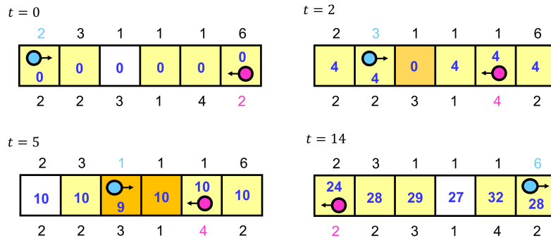
Obrázek 2: Schémata zachycující průběh průchodu robotů chodbou postupně v časech 0, 2, 5 a 14. Platí N = 6 , D_1 = 1 , D_2 = 2 . Úseky jsou reprezentovány čtverečky, první robot světle modrým kolečkem, druhý robot červeno-fialovým kolečkem. Úsek osvětlený jedním robotem je zvýrazněn žlutě, úsek osvětlený oběma roboty oranžově. Časy T_k jsou uvedené nad úseky, časy S_k pod úseky. Tmavě modrá čísla uvnitř úseků odpovídají doposud dosažené kvalitě osvětlení. Roboty dokončí pohyb v čase 14.
