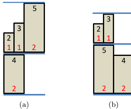
Obrázek 10: Knihovna s abecedně seřazenými knihami. Modré úsečky znázorňují police, béžové obdélníky knihy. Černé číslo v obdélníku je výška příslušné knihy, červené číslo je její tloušťka. Knihy v abecedním pořadí mají rozměry (výška \times tloušťka): 2 \times 1 , 3 \times 1 , 5 \times 2 , 4 \times 2 . Délka police je L = 4 . (a) Rozmístění knih podle naivního algoritmu s cenou 5 + 4 = 9 . (b) Jediné optimální řešení s cenou 3 + 5 = 8 a maximální mezerou 2.
